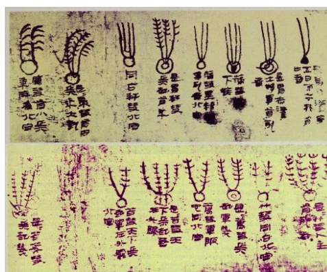
Fot. 2. Kształty głów i ogonów komet uwiecznione przez chińskiego astronoma ok. III wiek p.n.e.
